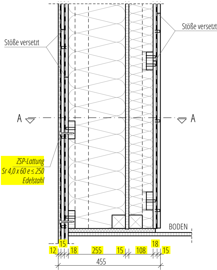
VERTIKALSCHNITT B - B
