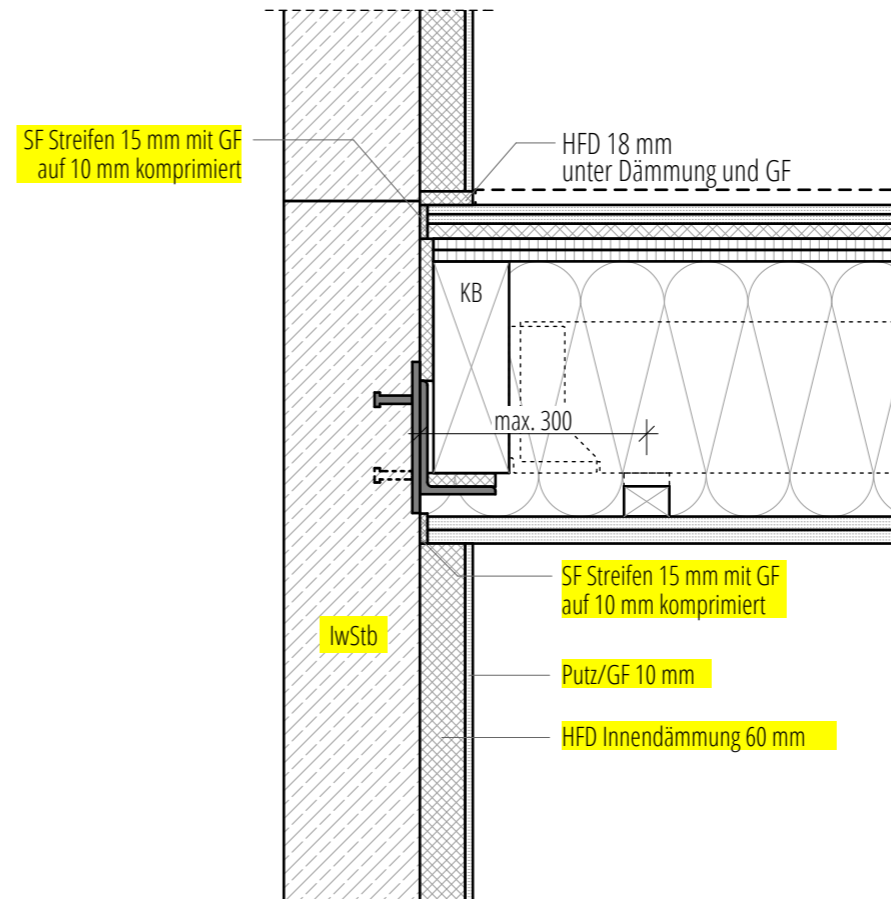
VERTIKALSCHNITT INNENWAND
