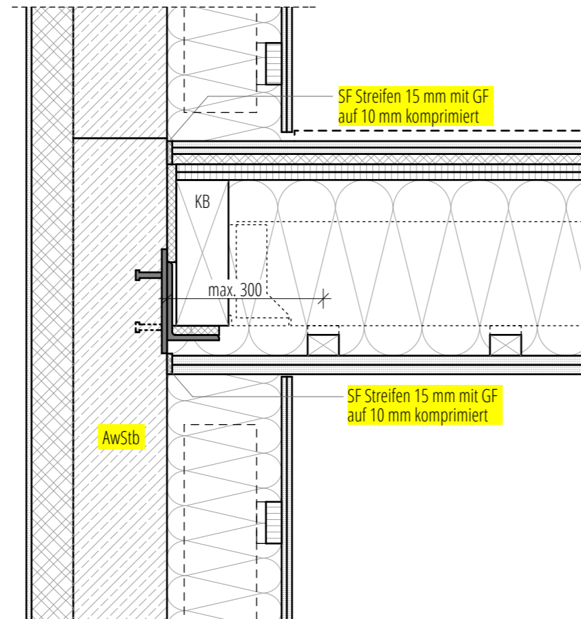
VERTIKALSCHNITT AUßENWAND
