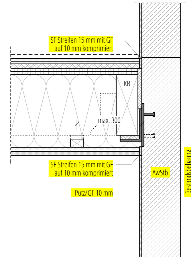
VERTIKALSCHNITT AUßENWAND NEBEN BESTANDSBEBAUUNG
