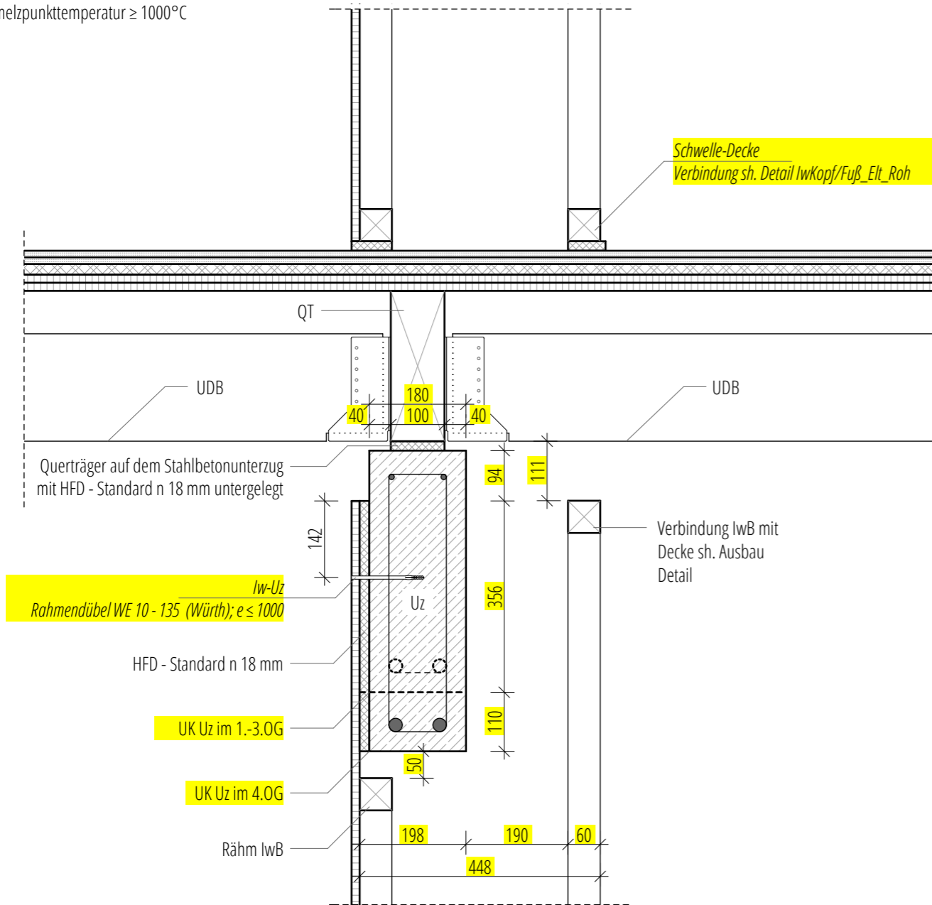
INNENWAND TYP B - INSTALLATIONSWAND
