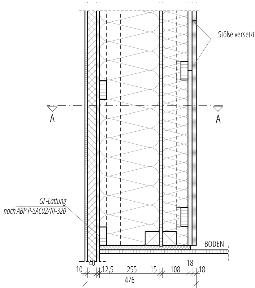
VERTIKALSCHNITT B - B
