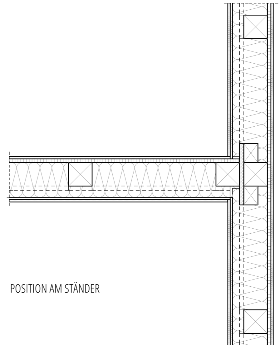
SITUATION 2: OSB GEGENÜBER DER SEITE DER ANGESCHLOSSENEN INNENWAND
