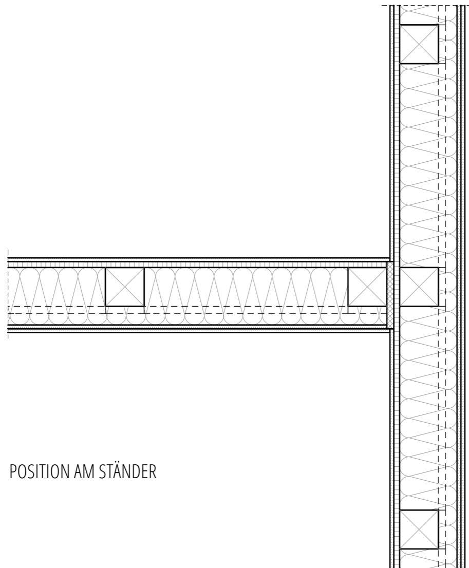
SITUATION 1: OSB AUF DER SEITE DER ANGESCHLOSSENEN INNENWAND
