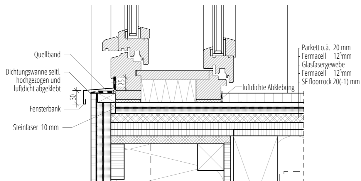
UNTEN - FENSTERTÜR
