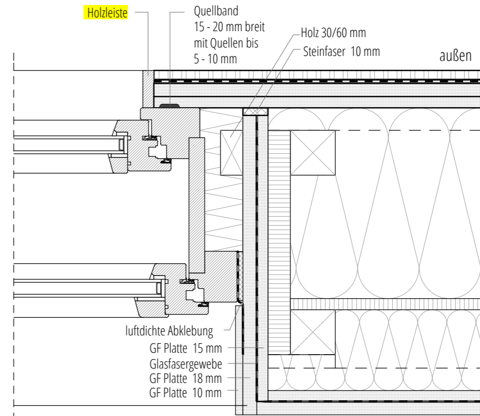
SEITE - BRÜSTUNGSFENSTER / FENSTERTÜR
