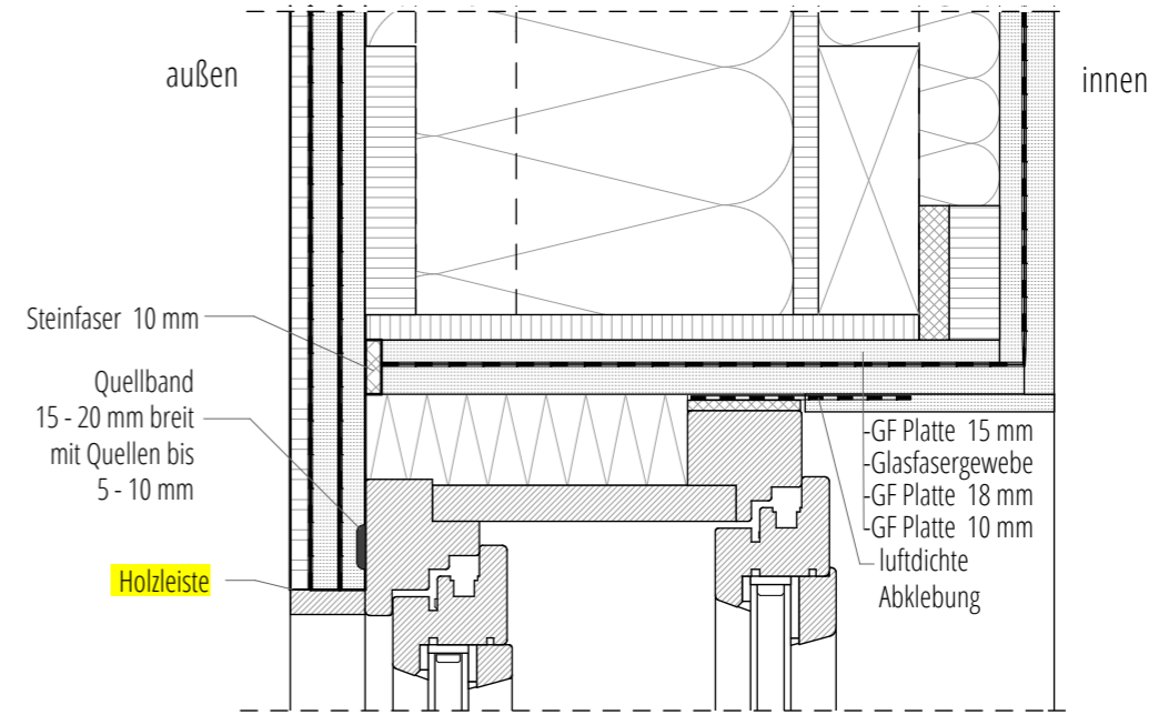
OBEN - MIT FENSTERSTURZ
