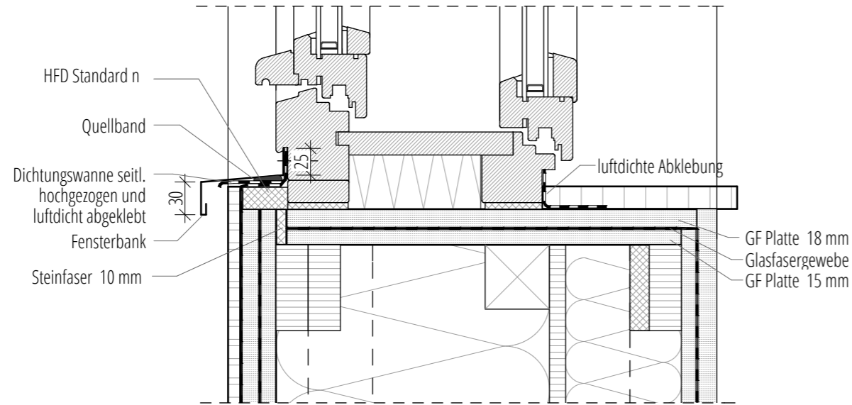
UNTEN - BRÜSTUNGSFENSTER
