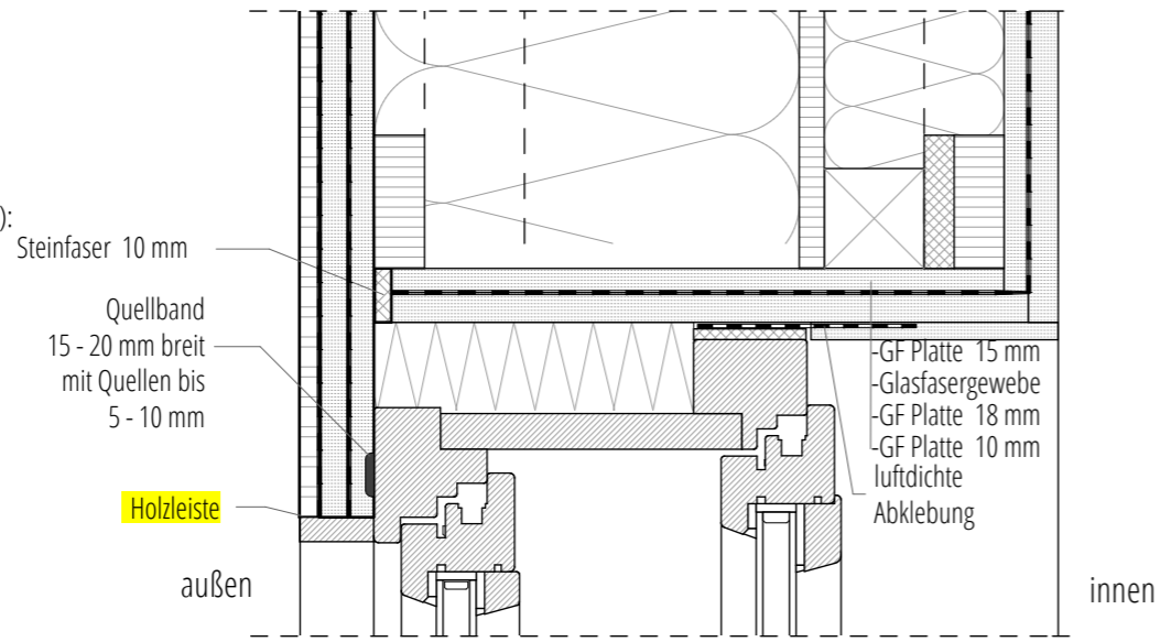
OBEN - OHNE FENSTERSTURZ
