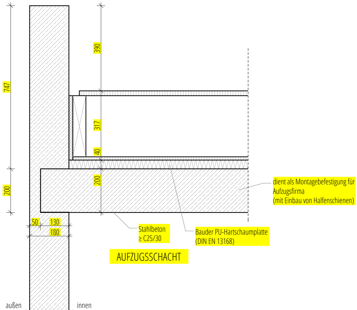
ANSCHLUSSSITUATION AM ORTGANG
